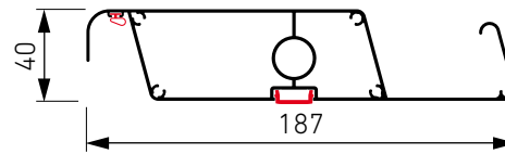
P-190 LED slat ■ 050189
