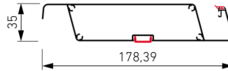
P-150 LED slat ■ 050210
